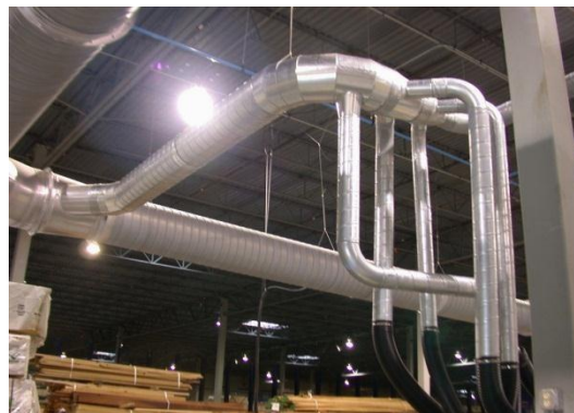
transporte neumático(colectores de aserrín) 2011 Feicobol
